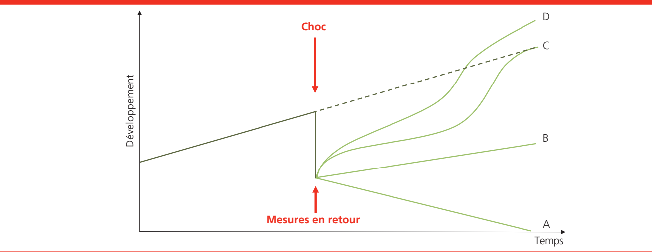
Figure 2 les différents effets d'un choc, source : d'après Mitchel & Harris, 2012
