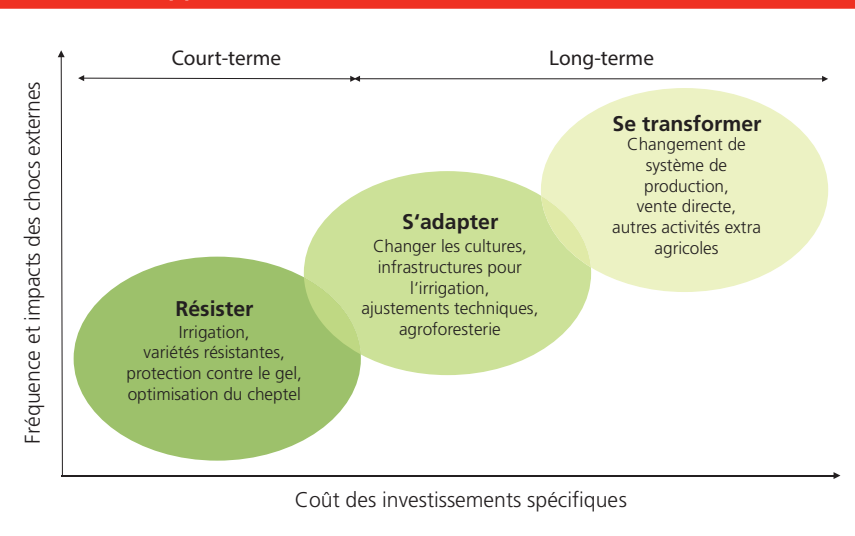
Figure 1 les 3 stratégies en réponse à un choc extrême, d'après Sylvain Pellerin, INRA (F)
