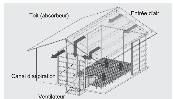
FIGURE 3 : Schéma d'une installation avec séchage solaire.
