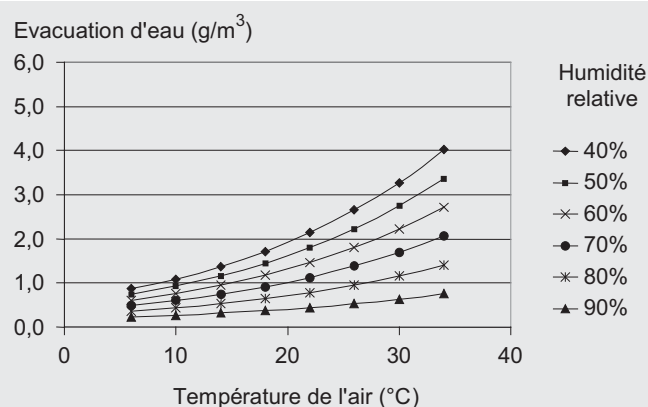
FIGURE 1 : Influence de la température et de l'humidité relative de l'air sur l'évacuation effective de l'eau pour un fourrage avec une teneur en matière sèche de 70%.
